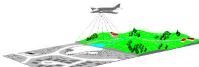
Abb.1: Meßprinzip Laserscanner (TopoSys)
